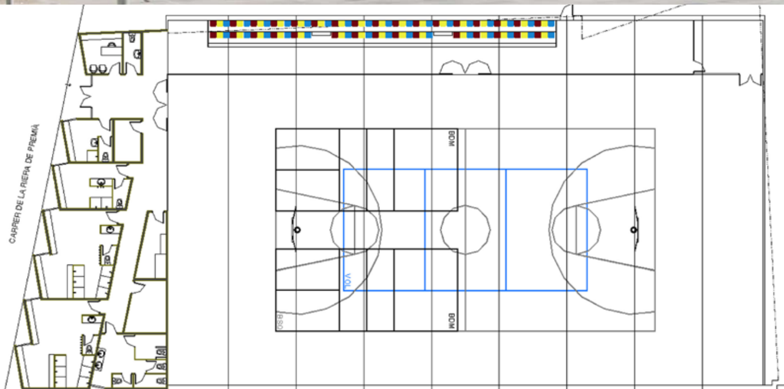
A dalt, estat actual de la pista del Voramar. A baix, plànol del futur pavelló que s'hi construirà
