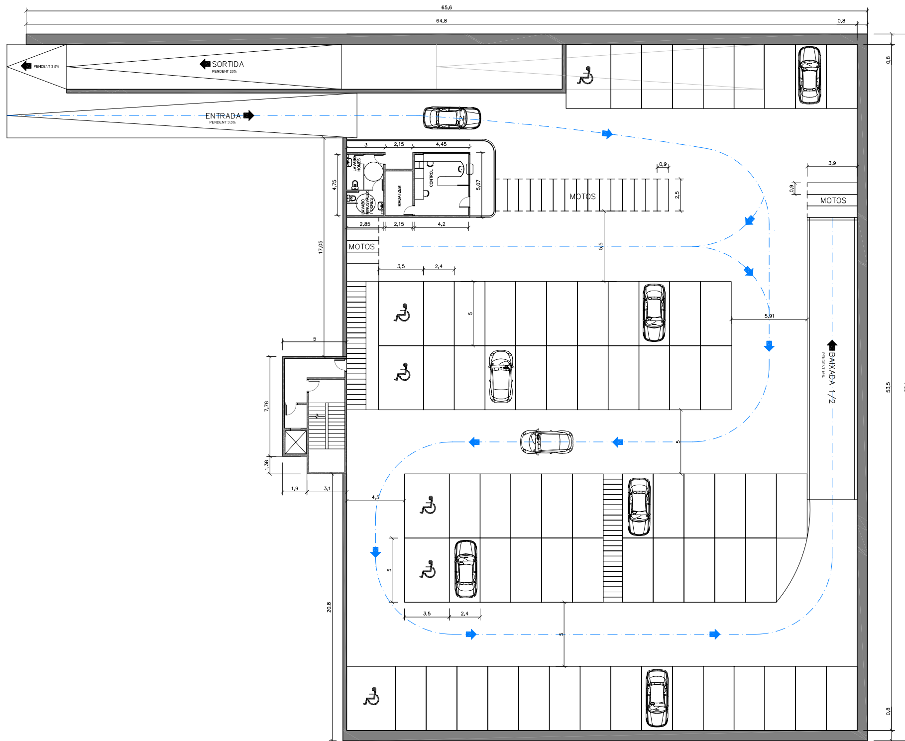
PLANTA -1 COTES
