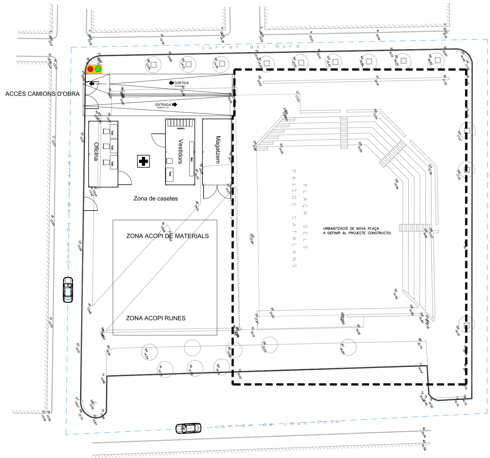
PLANTA PLAÇA
